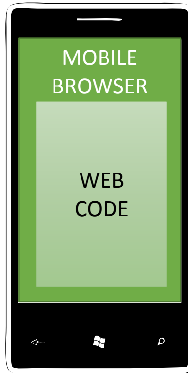
Web-Application
